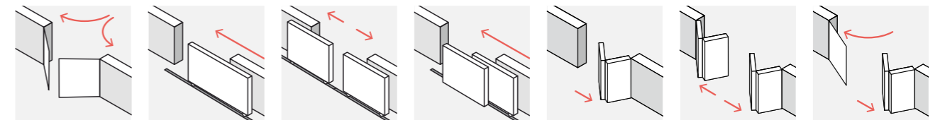
Battant (ouverture jusqu'à 180°) Coulissant Double coulissant (double motorisation) Télescopique (portails pleins et droits) Battant repliable (portails droits et motorisés, 1 vantail) Battant repliable (portails droits et motorisés, 2 vantaux) Battant et battant repliable (portails droits et motorisés, 1 vantail de chaque)
